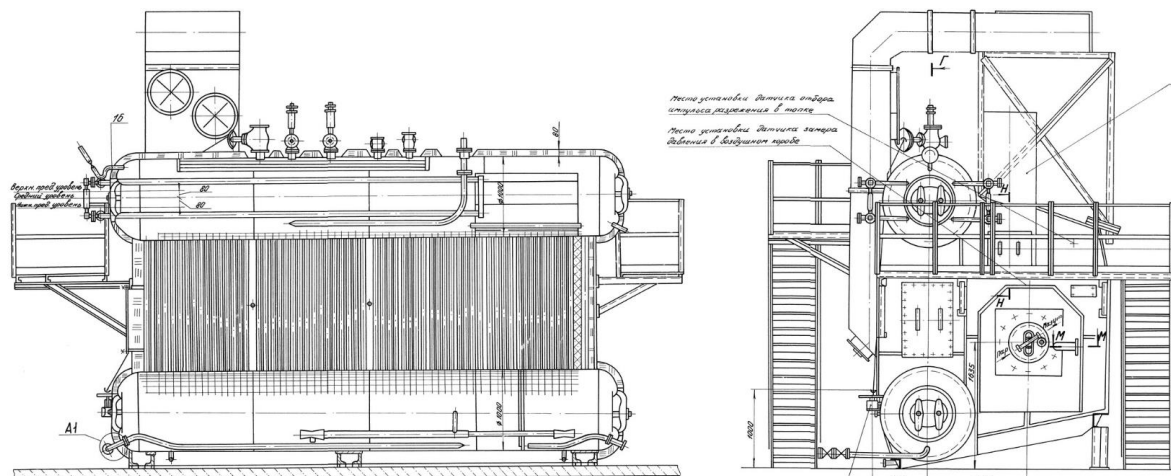
Рис. 11 Общий вид котла ДЕ 10-14
