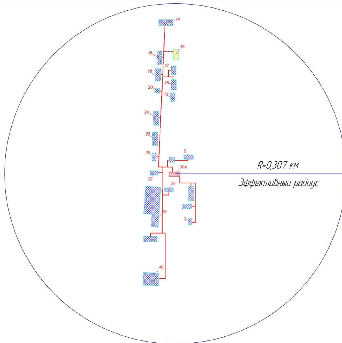
Рис 21. Радиус эффективного действия Котельной №3.
